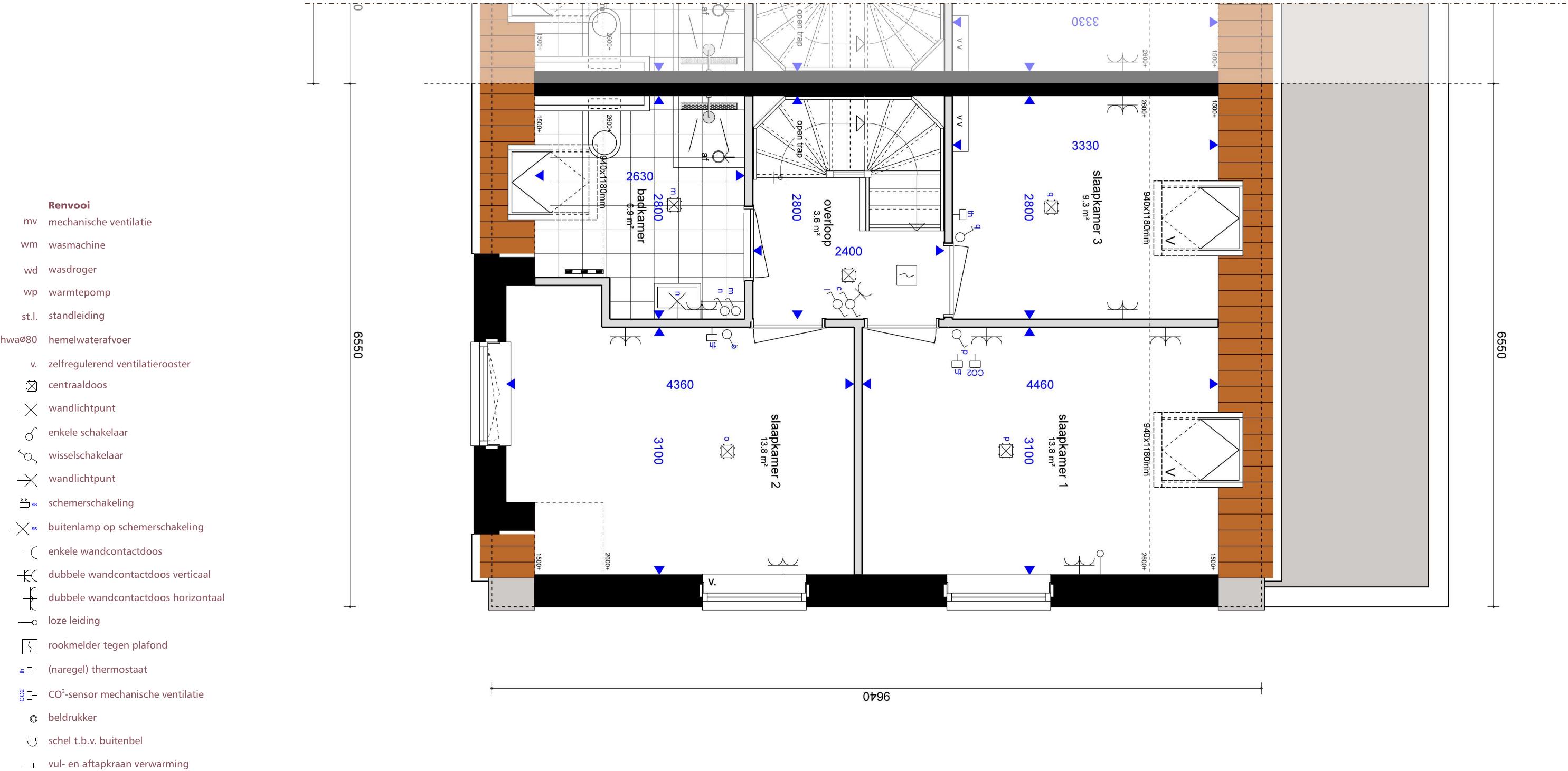
SCHAAL 1 OP 50 Plattegrond ~ Eerste verdieping
